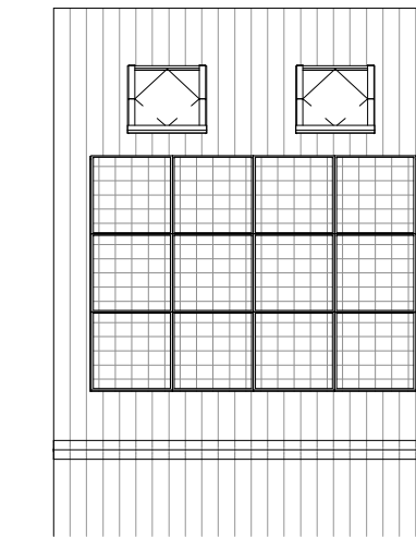
Dak plattgrond
